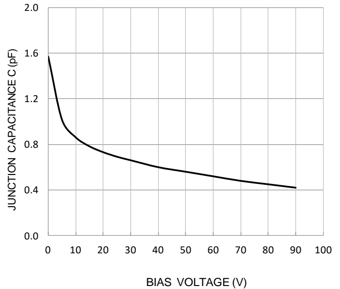
逆特性 (代表例)
