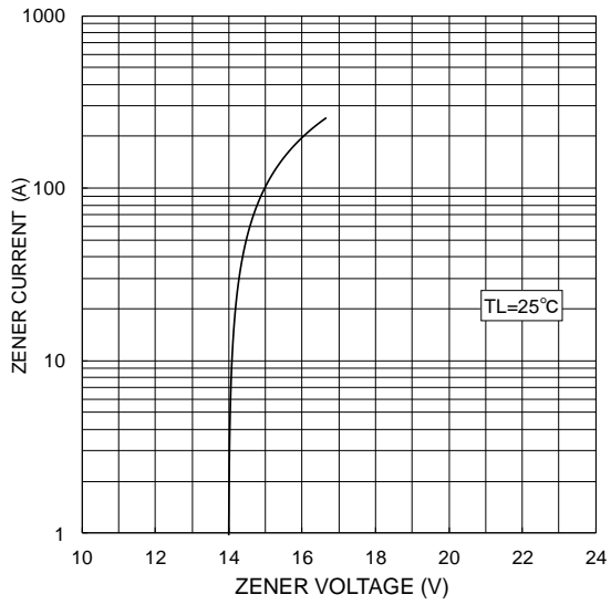
ツェナー特性 (代表値) Typical zener characteristics
