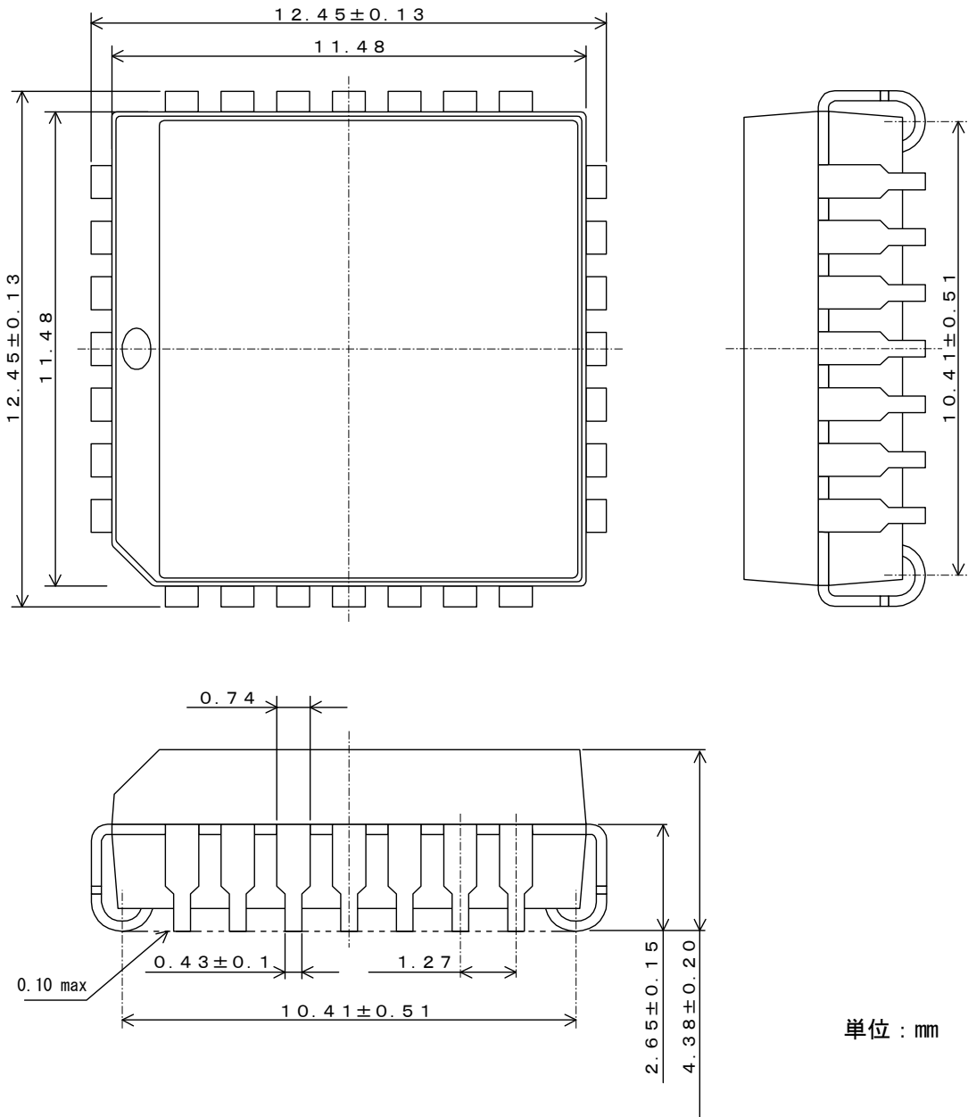
図4. 外形寸法図
