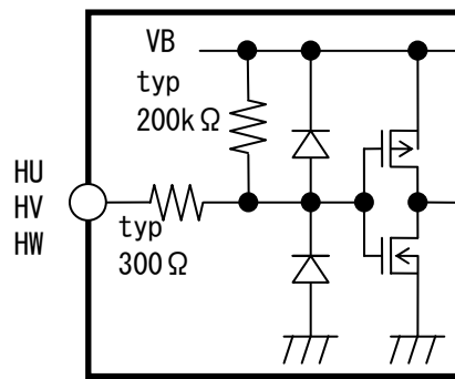
図 1. HU, HV, HW 端子の等価回路
