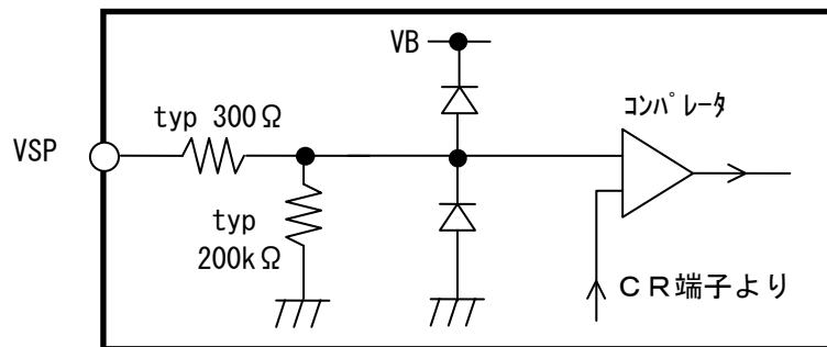
図 2. VSP 端子の等価回路
