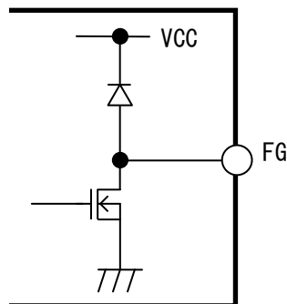
図 3. FG 端子の等価回路
