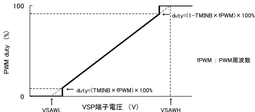
図5. PWM dutyとVSP入力電圧の関係
