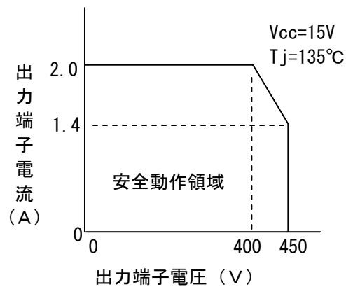
図6. 安全動作領域
