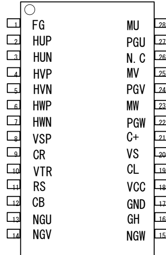
(上面図)
