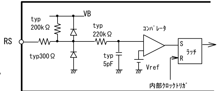
図 2.2.1 RS 端子の等価回路
