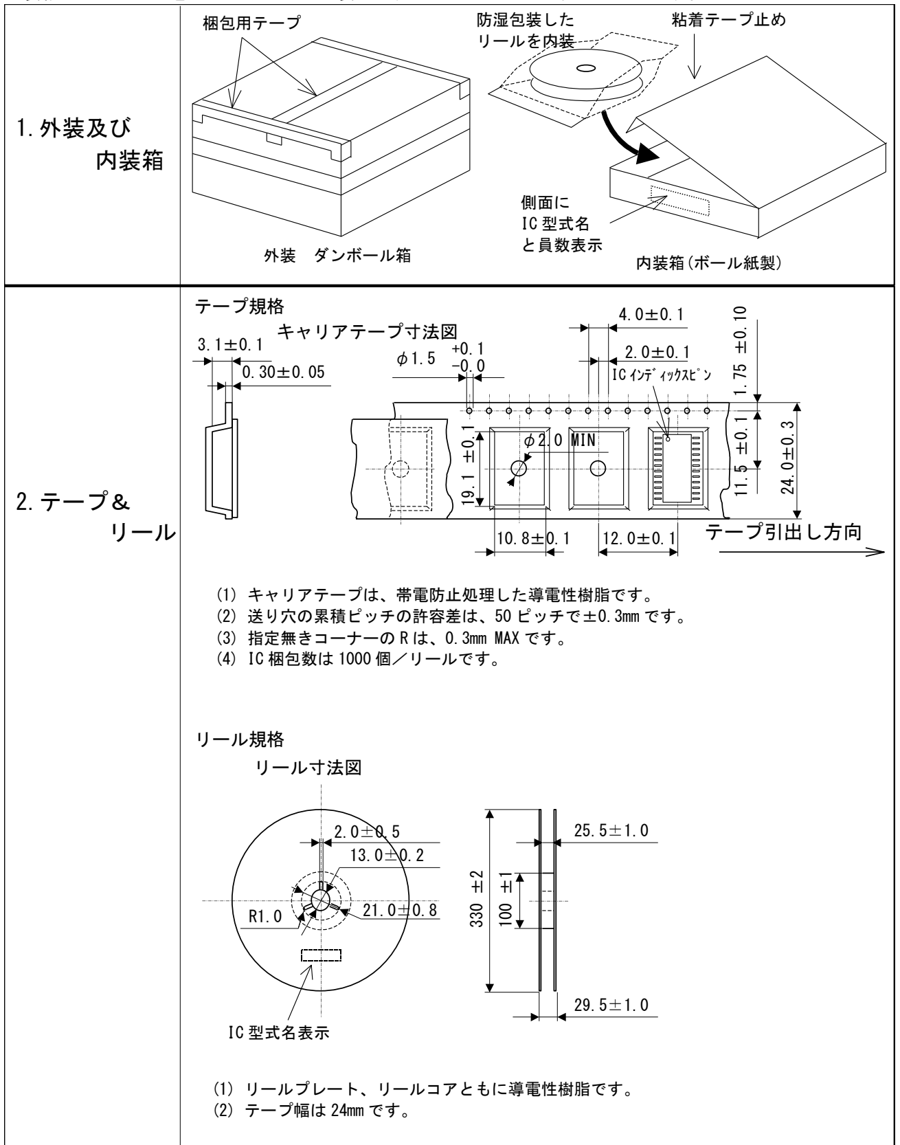
図9.3.1 梱包形態
