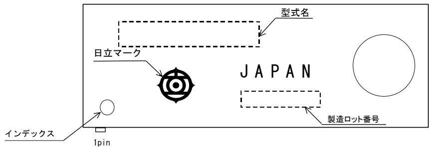
図9.2.1.1 マーク位置
