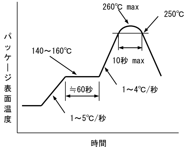
図7.6.1 赤外線リフローおよびエアリフロー推奨条件
