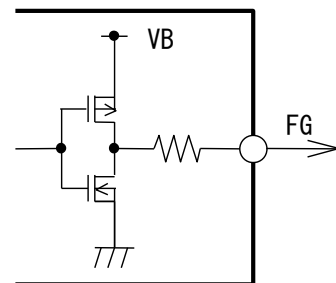
図 2.2.3 FG 端子の等価出力回路
