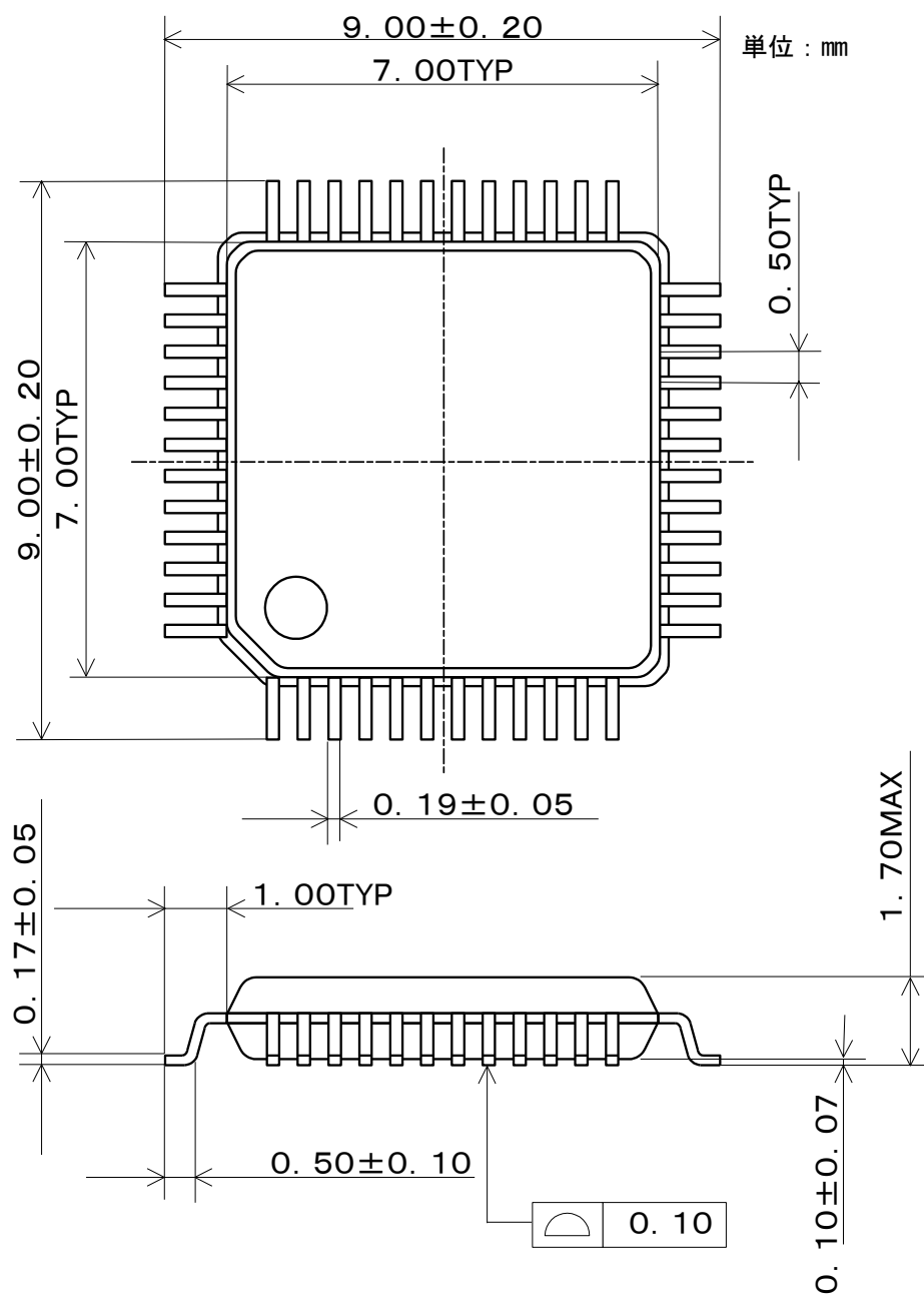
図 6. 外形寸法図
