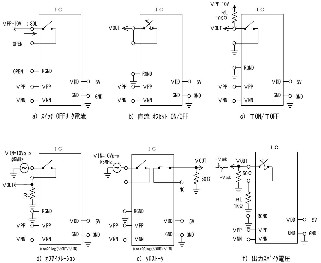
図2. 測定回路
