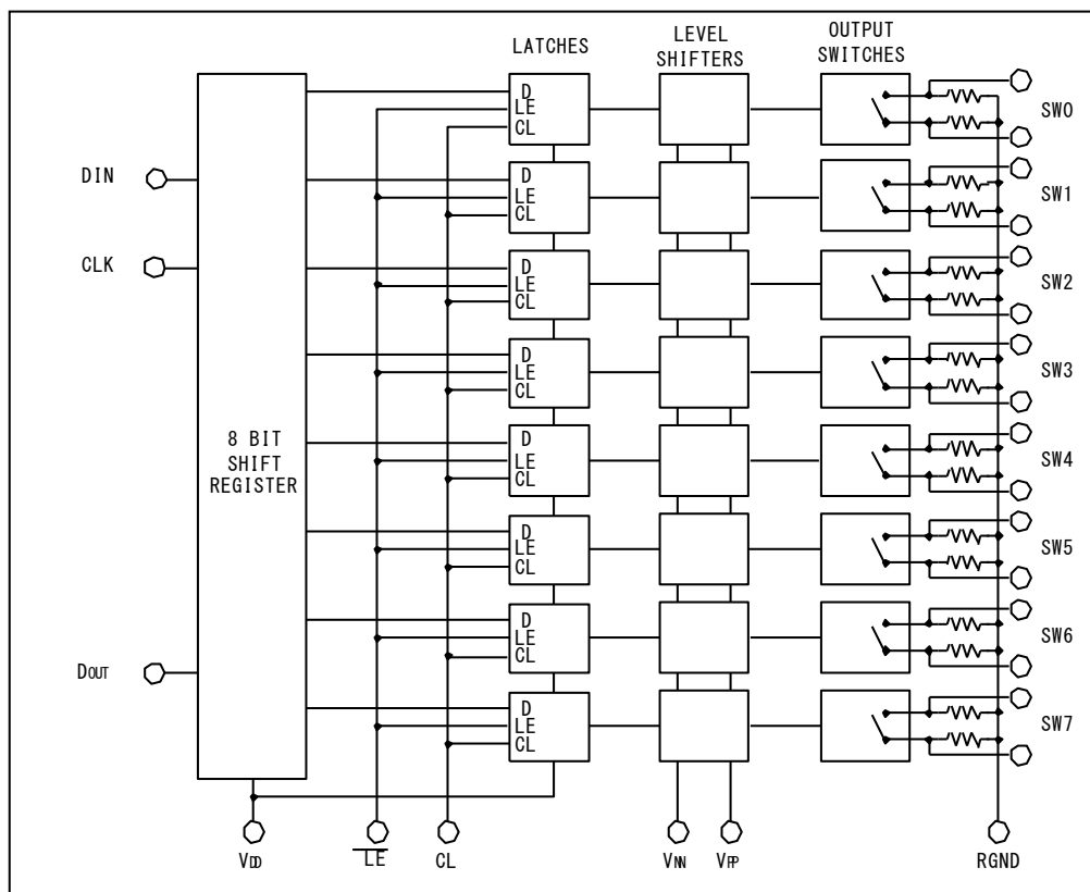
図 1. 回路ブロック図
