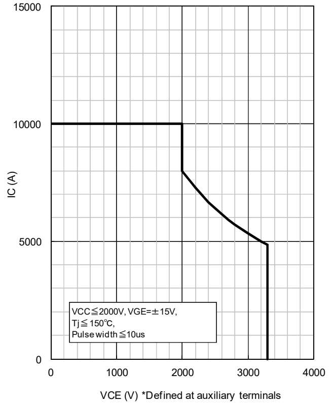
SCSOA
