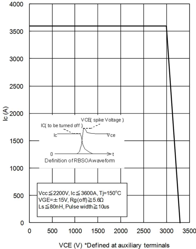
RBSOA
