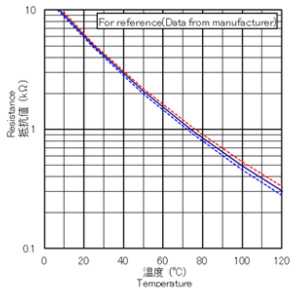
サーミスタ抵抗-温度特性 Thermistor Resistance-Temperature Characteristics
