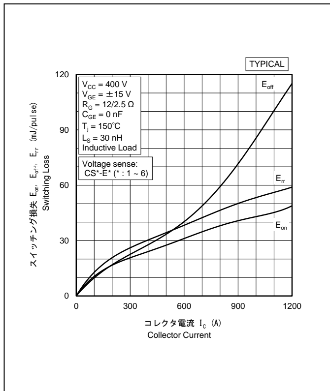
スイッチング損失-コレクタ電流特性 Switching Loss-Collector Current Characteristics
