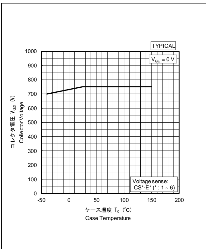
主耐圧特性 (温度依存性) Collector Emitter Voltage vs. Case Temperature
