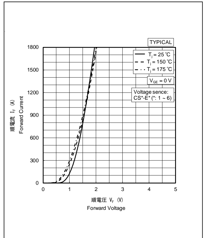
フリーホイールダイオード順電圧特性 Forward Voltage of Free-Wheeling Diode
