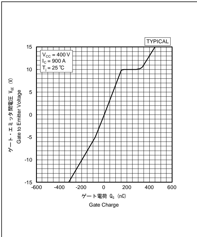
ゲート電荷特性 Gate Charge Characteristics
