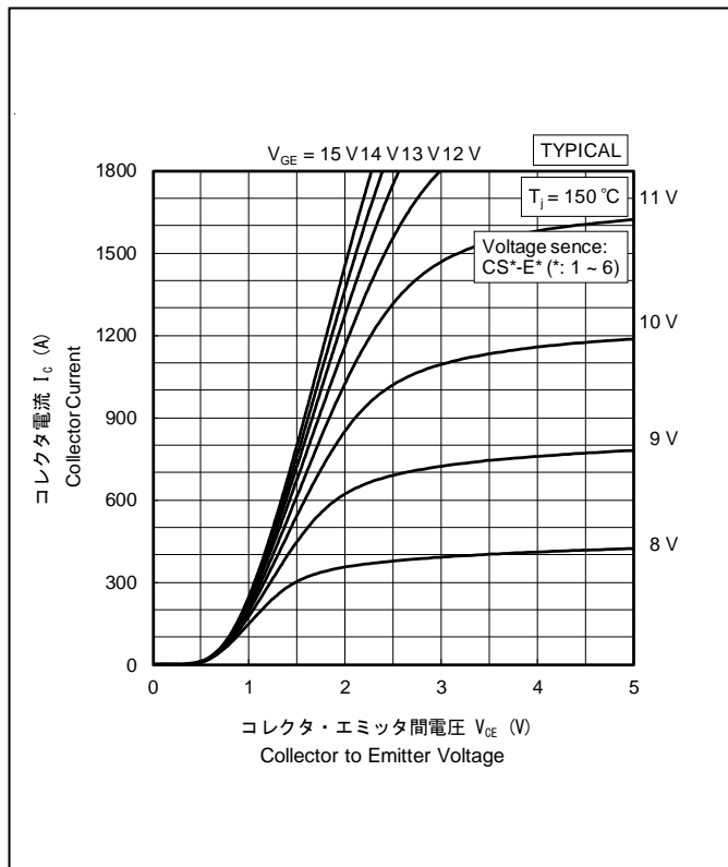
コレクタ電流—コレクタ・エミッタ間電圧特性 (150 °C) Collector Current vs. Collector to Emitter Voltage (150 °C)
