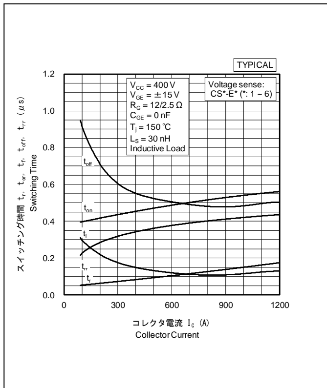
スイッチング時間-コレクタ電流特性 Switching Time-Collector Current Characteristics
